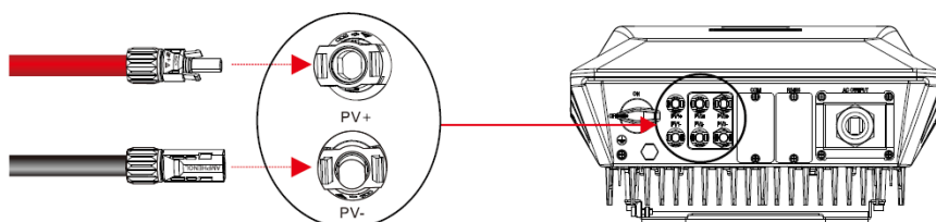
Fig. 20: Connessione dei cavi assemblati all'inverter SMT
