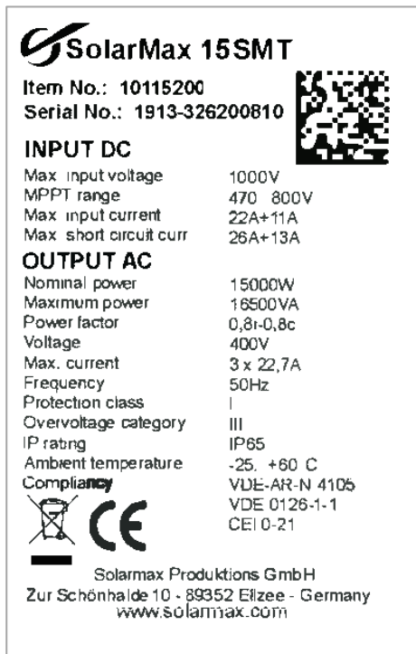
Fig. 1: Targhetta prodotto del SolarMax 15SMT
