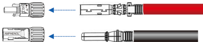
Fig. 17: Inserimento dei puntali crimpati nel corpo del connettore
