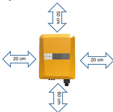
Fig. 5: Distanze minime di rispetto inverter SMT
