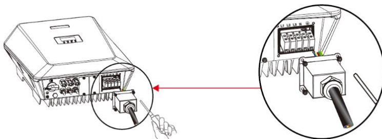
Fig. 12: Fissaggio della copertura stagna
