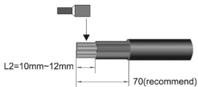
Fig. 8: Rimozione dell'isolamento dal cavo AC
