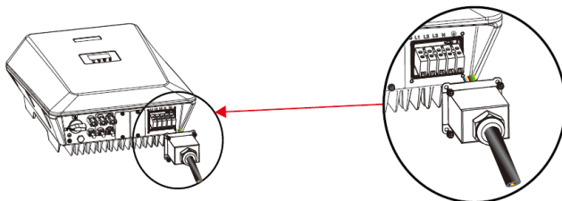
Fig. 10: Preparazione del cavo AC per la connessione
