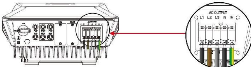
Fig. 11: Collegamento dei conduttori
