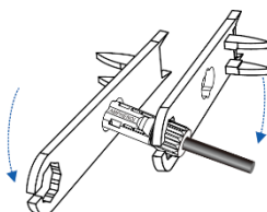
Fig. 18: Serraggio del dado di bloccaggio
