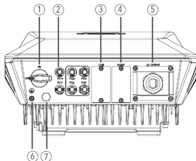
Fig. 4: Connessioni nella parte inferiore
